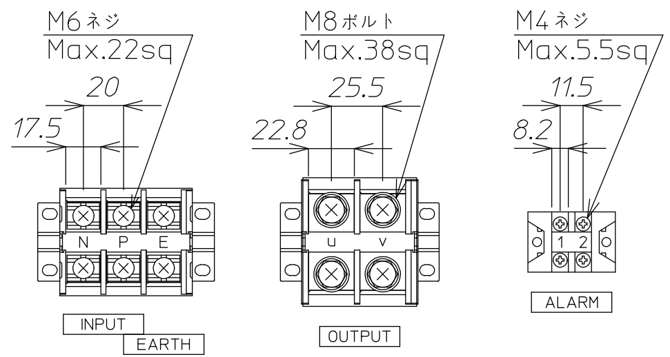
端子詳細図
